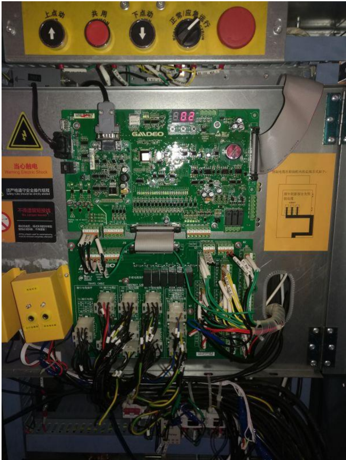
电梯控制柜 2
