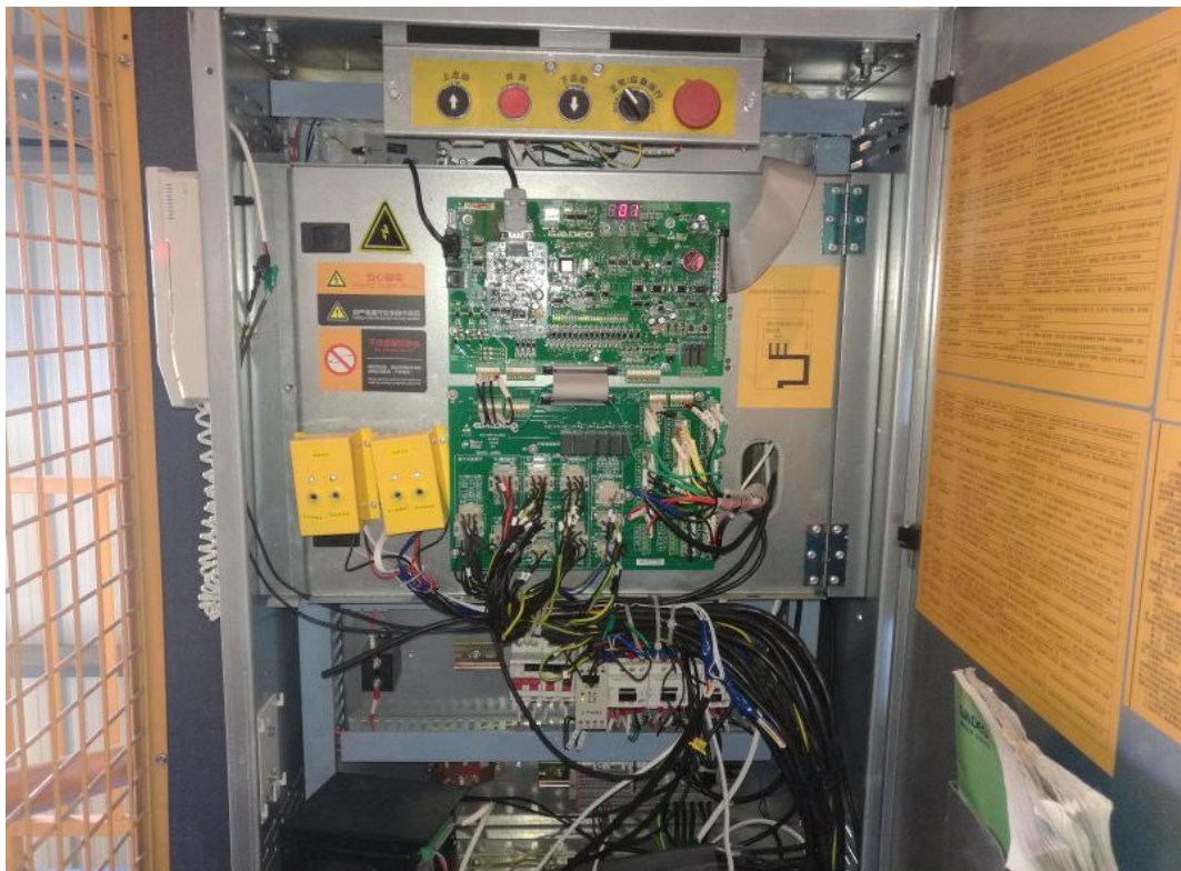
电梯控制柜 1
