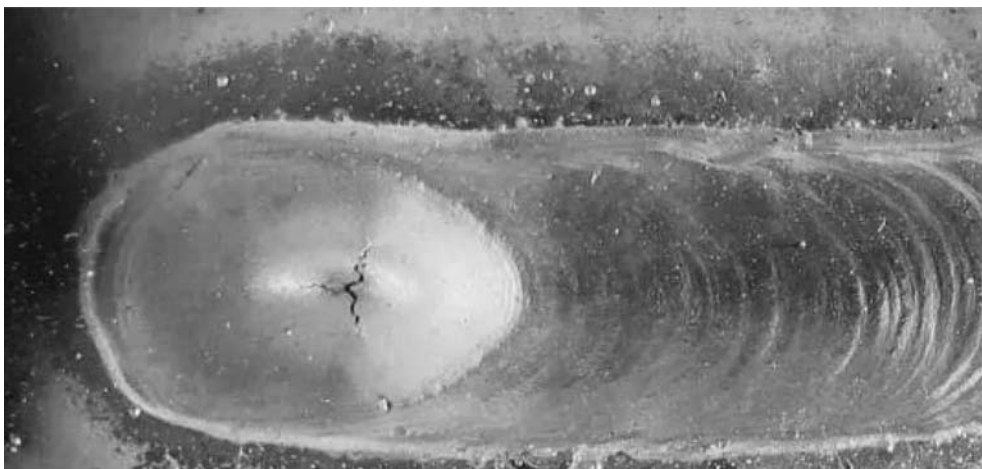
图 1 焊接裂纹
